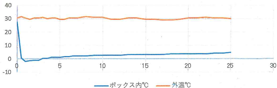
プレート6枚/保冷库内温度&外温
